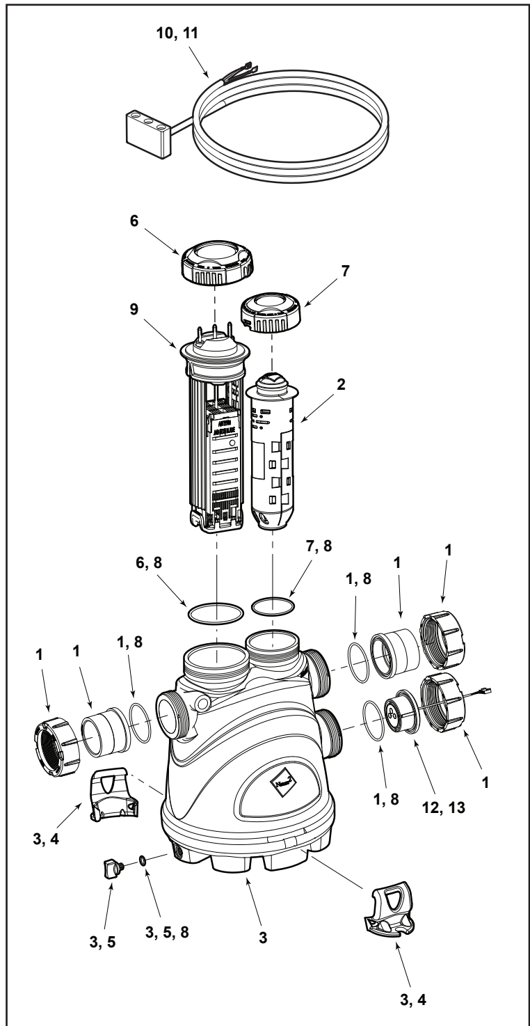
Figura 21. Vista ampliada del Nature 2 Fusion Soft
