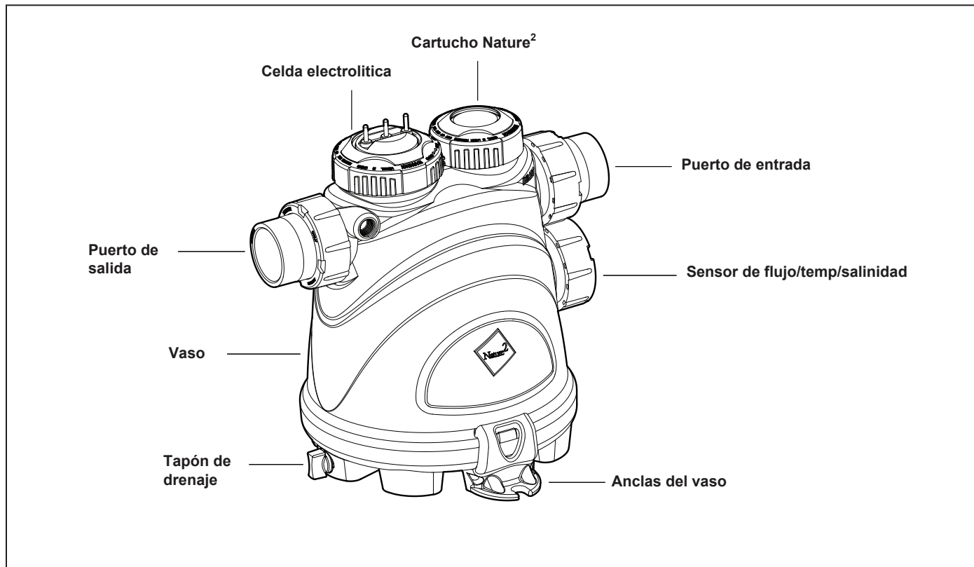
Figura 1. Componentes del Nature 2 Fusion Soft
